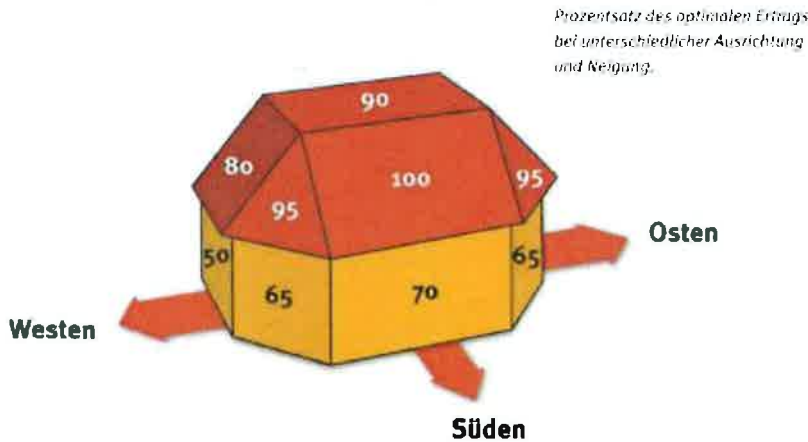
Abb. 4: Prozentsatz des optimalen Ertrags bei unterschiedlicher Ausrichtung und Neigung einer Dachflächen Quelle: Verbraucherzentrale Rheinland-Pfalz
